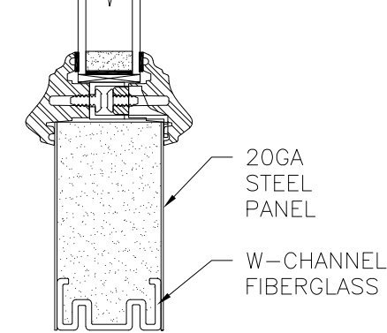
OPTION 26 PLUGLESS TRIM W/TAPE
