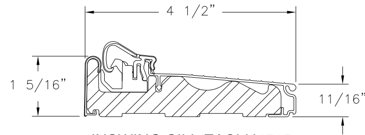
INSWING SILL ZAQLH4565
