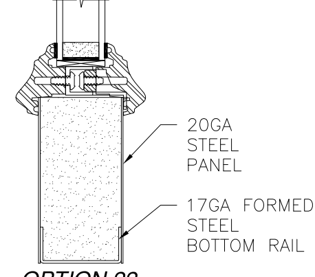
OPTION 22 PLUGLESS TRIM W/TAPE
