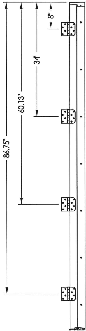
HINGE JAMB
