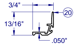
INTERLOCK S-2001
