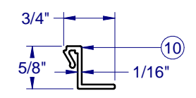
INTERLOCK S-2001
