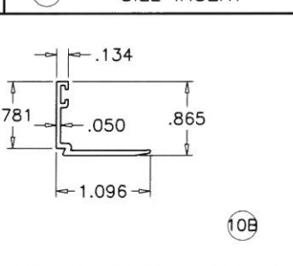
28 SILL INSERT
