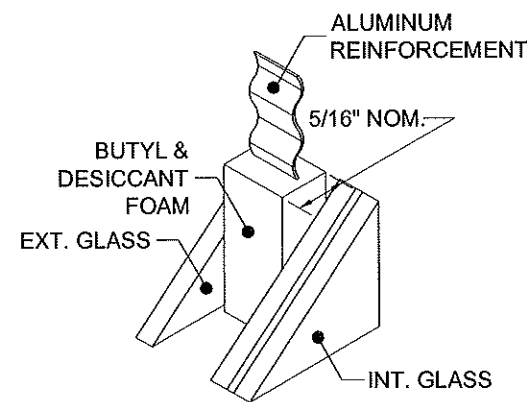
77 DURASEAL ® SPACER
