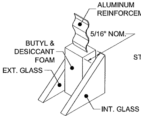
78 DURASEAL® SPACER
