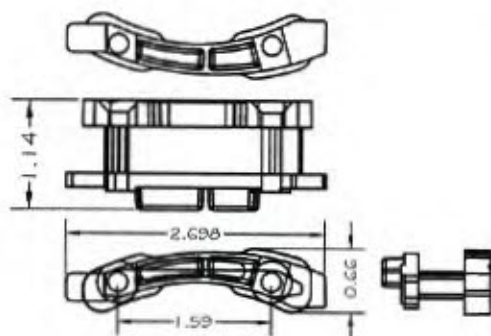
B- SLAT END LOCK ACETAL
