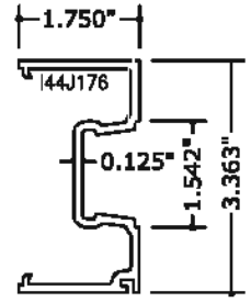
5 FRAME JAMB
