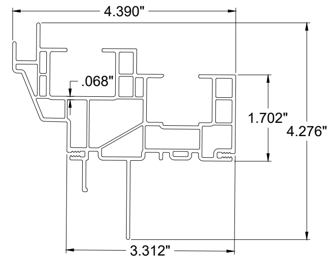
①C FIN/FLANGE FRAME
