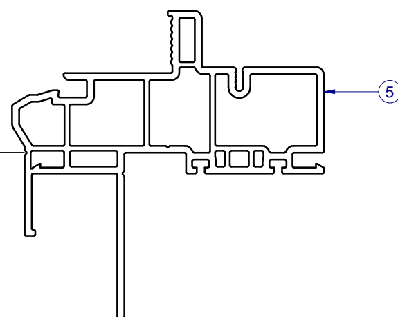
ALTERNATE FIN FRAME
