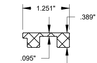
14 REINFORCEMENT (SASH STILE)
