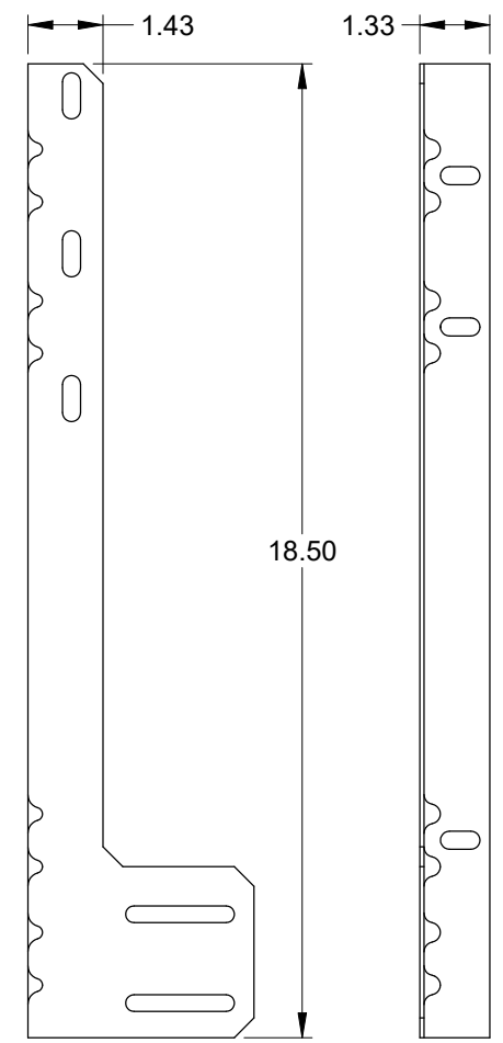
Jamb Angle .078 min. Galv. Steel
