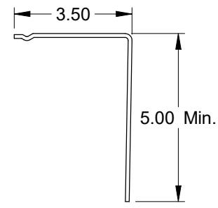
3" Angle Mount (Opt.) .086 Min. Galv. Steel
