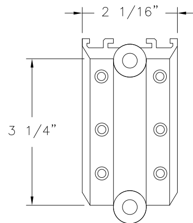
⑪ HINGE ALUMINUM 6063-T5
