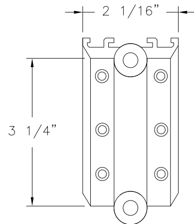
⑪ HINGE ALUMINUM 6063-T5
