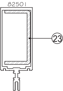
MULLION (J2)
