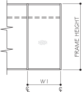
WIDTH (W) = W1 (JAMB)
