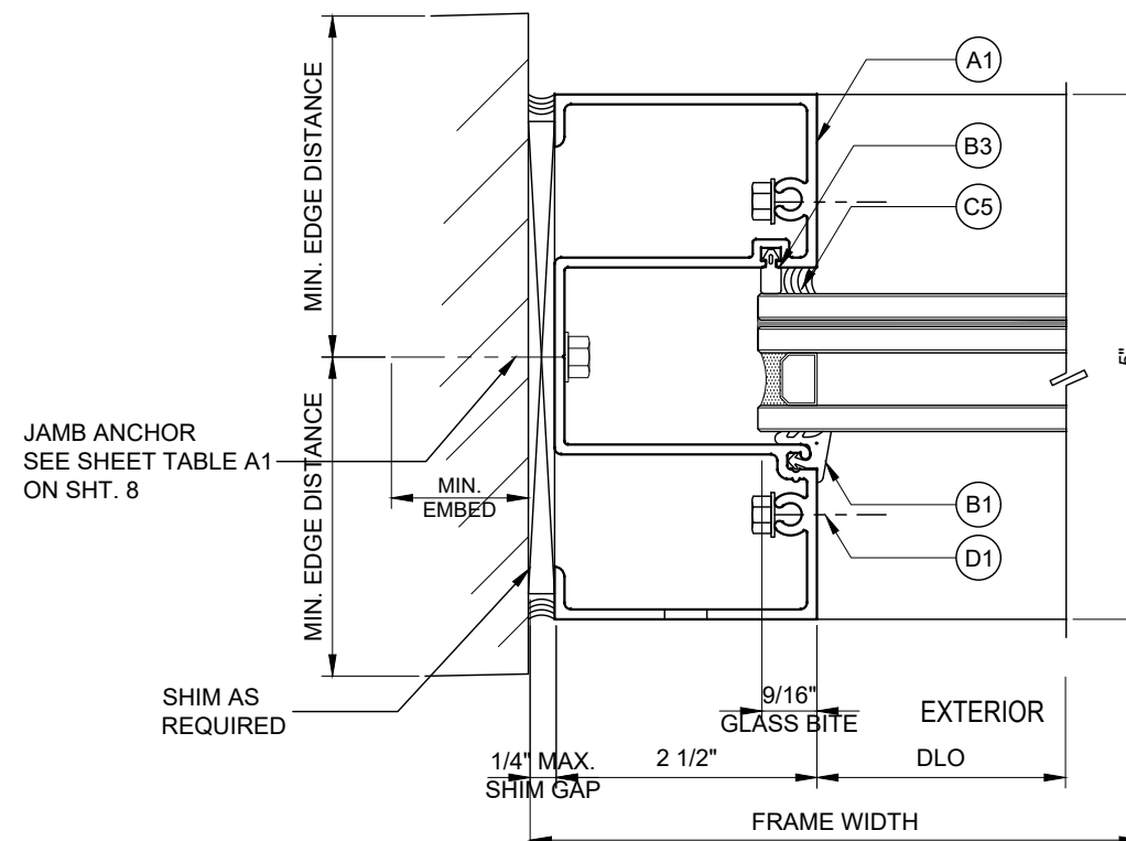
3 JAMB
