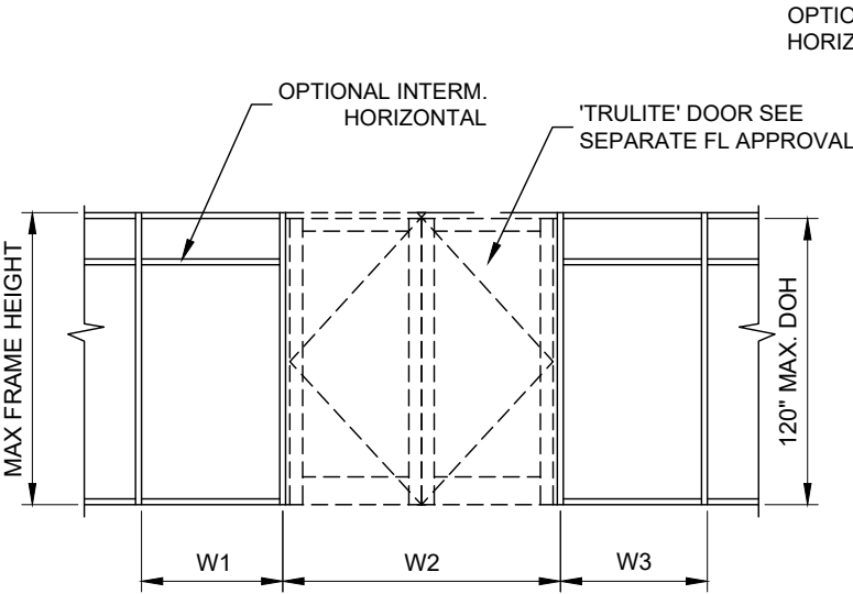
ELEVATION E2
