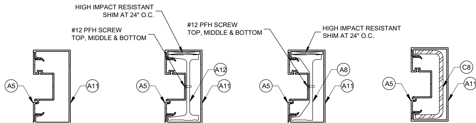
ELEVATION E5
