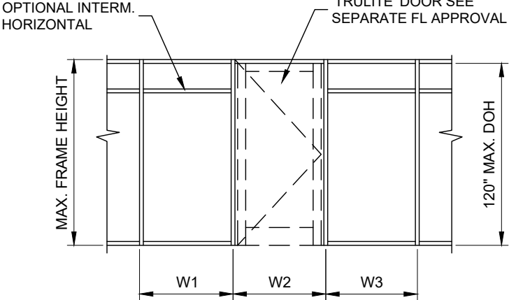
ELEVATION E4
