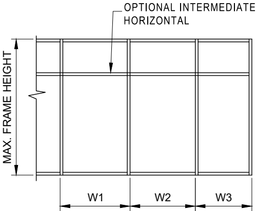
ELEVATION E1
