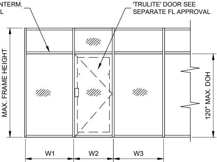
ELEVATION E3
