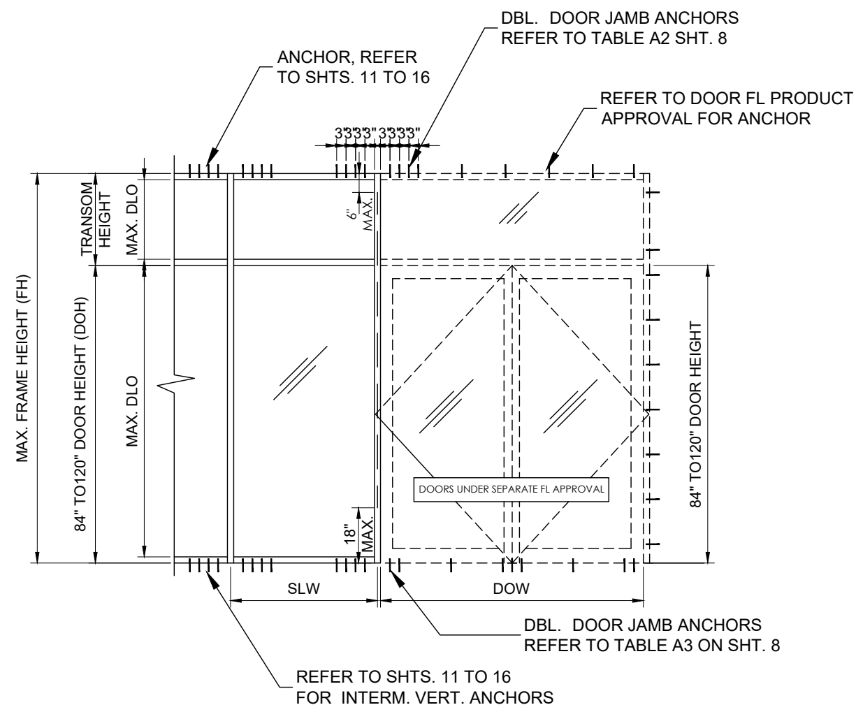
ELEVATION E5
