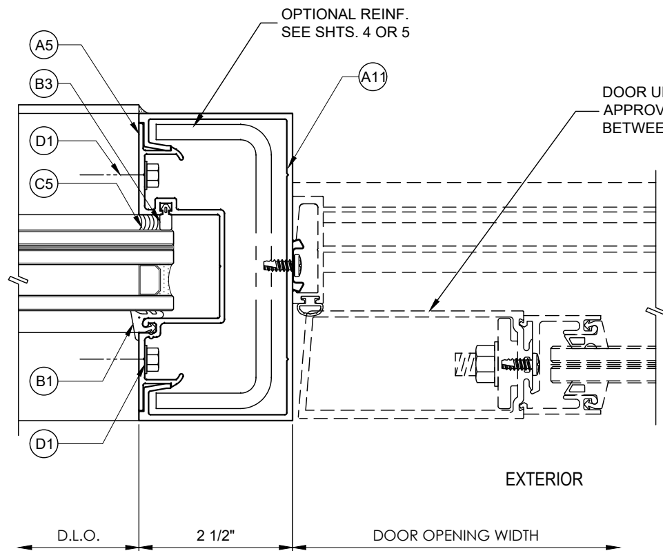
1 DOOR JAMB @ SIDELITE
