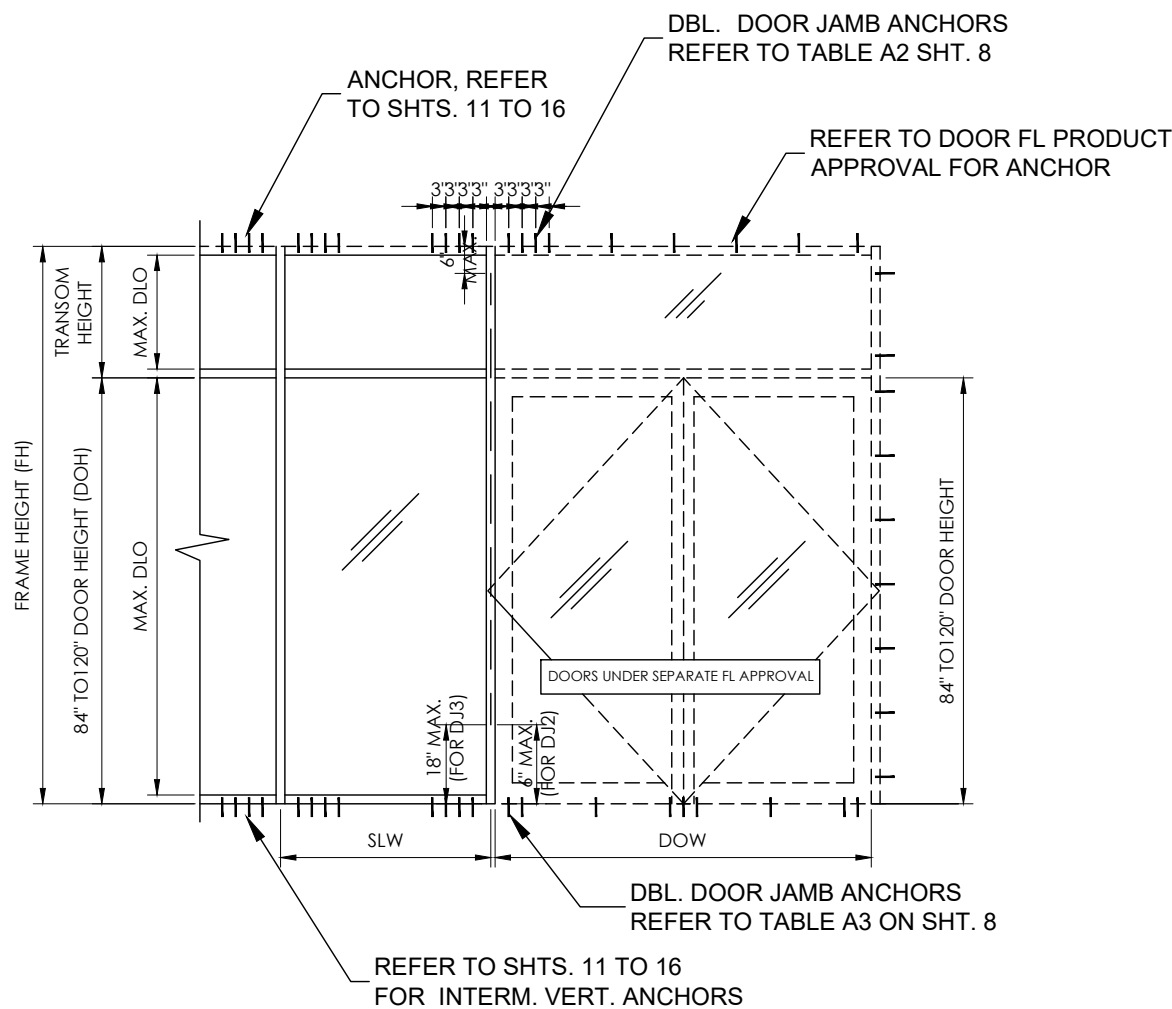
ELEVATION E5
