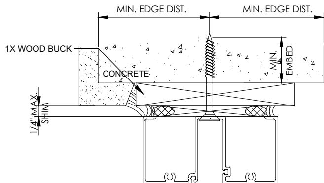
TYPE C, CC, D or DD
