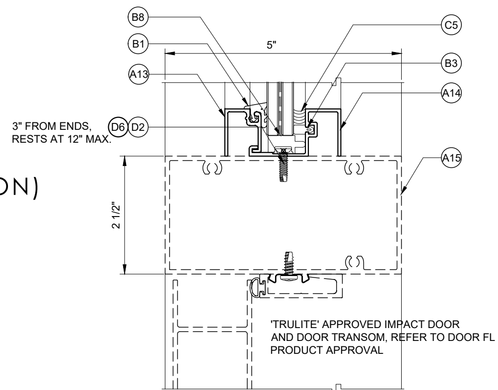
4 DOOR TRANSOM DETAIL
