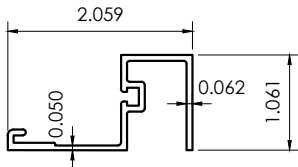
A14 TRANSOM SASH DF106
