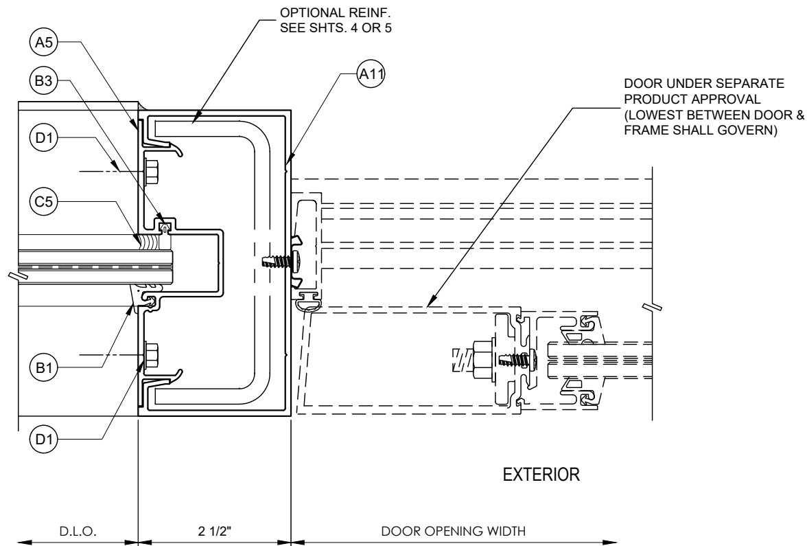
1 DOOR JAMB @ SIDELITE
