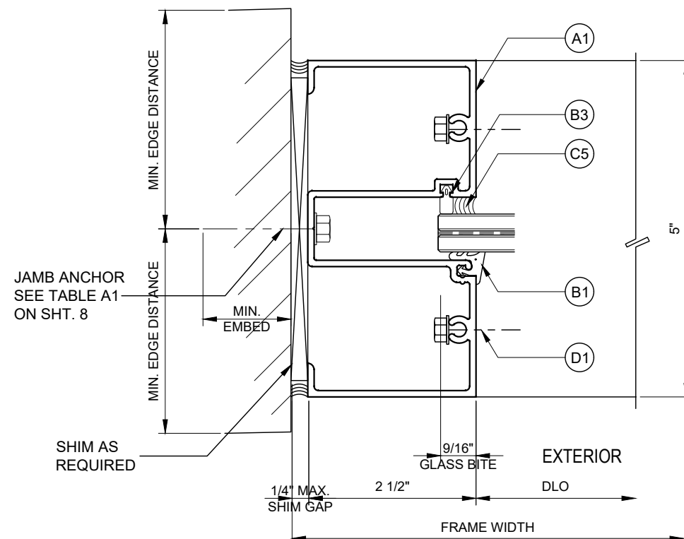
3 JAMB
