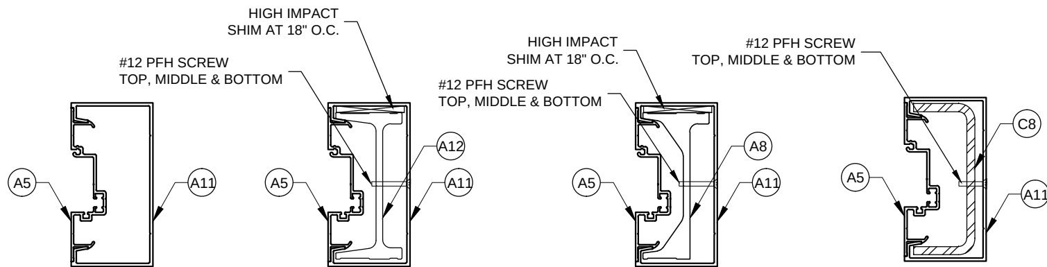
ELEVATION E5
