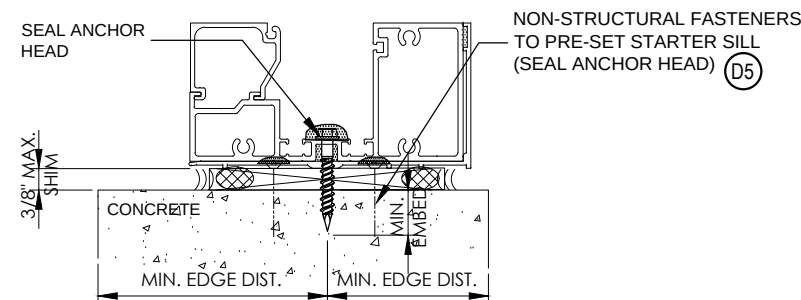
TYPES C, CC, D or DD
