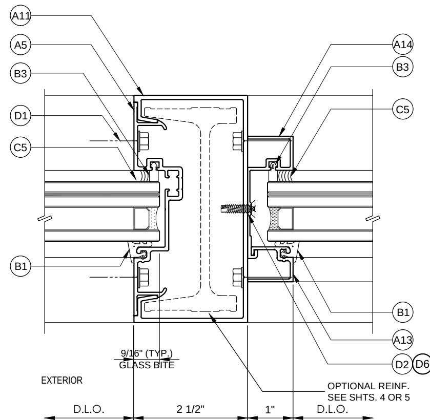
1 DOOR JAMB @ SIDELITE
