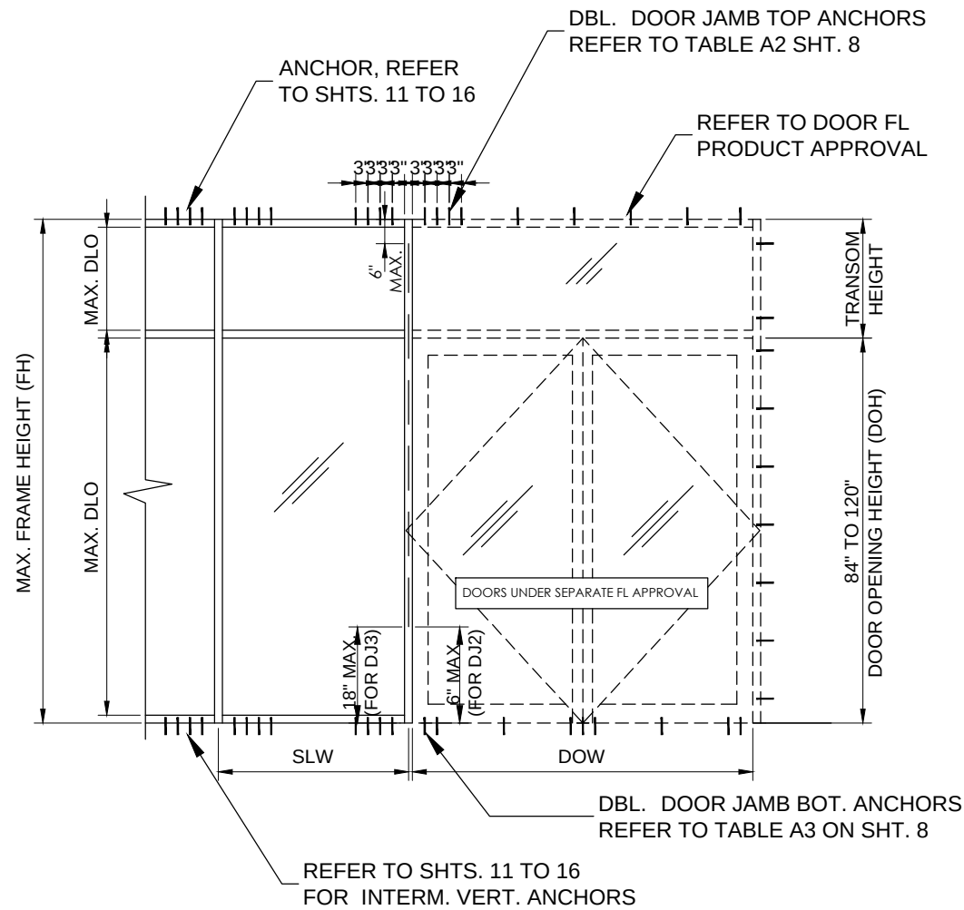
ELEVATION E5
