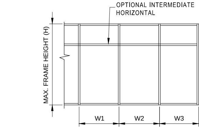
ELEVATION E1
