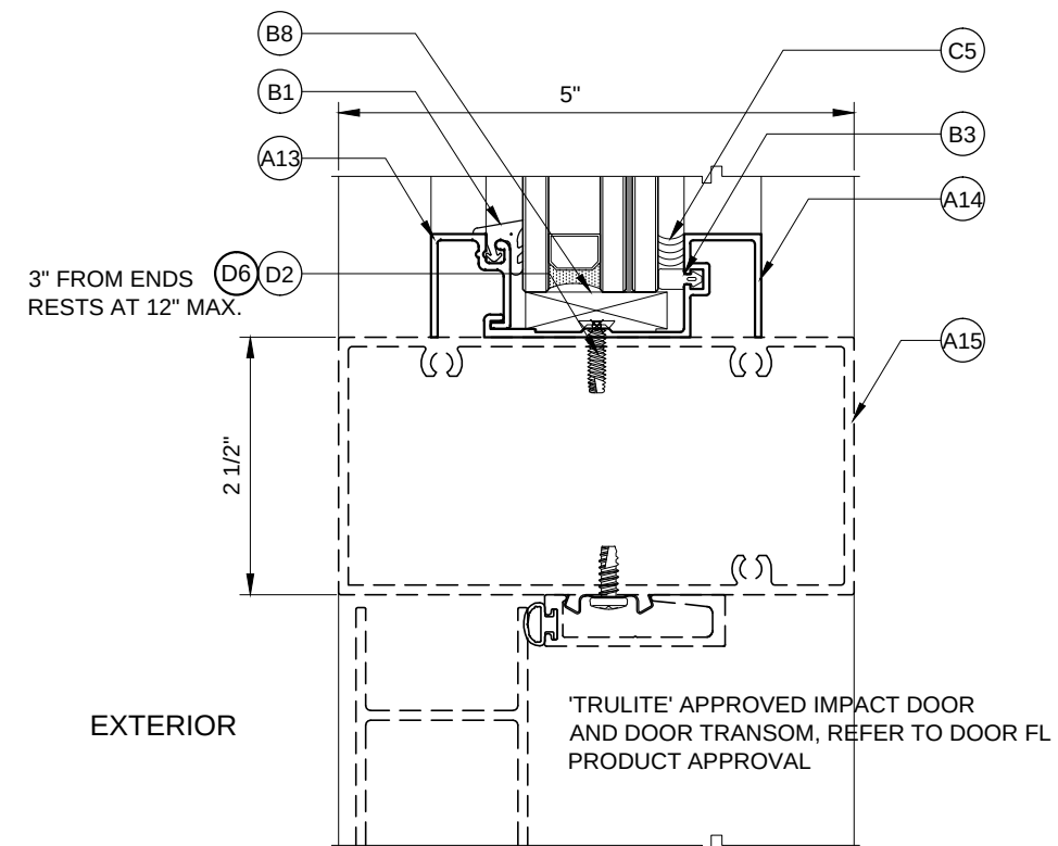
3 DOOR TRANSOM DETAIL
