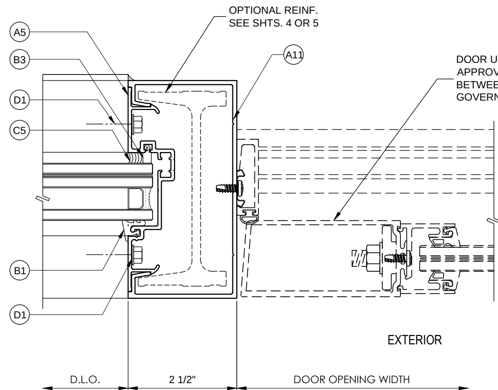
1 DOOR JAMB @ SIDELITE
